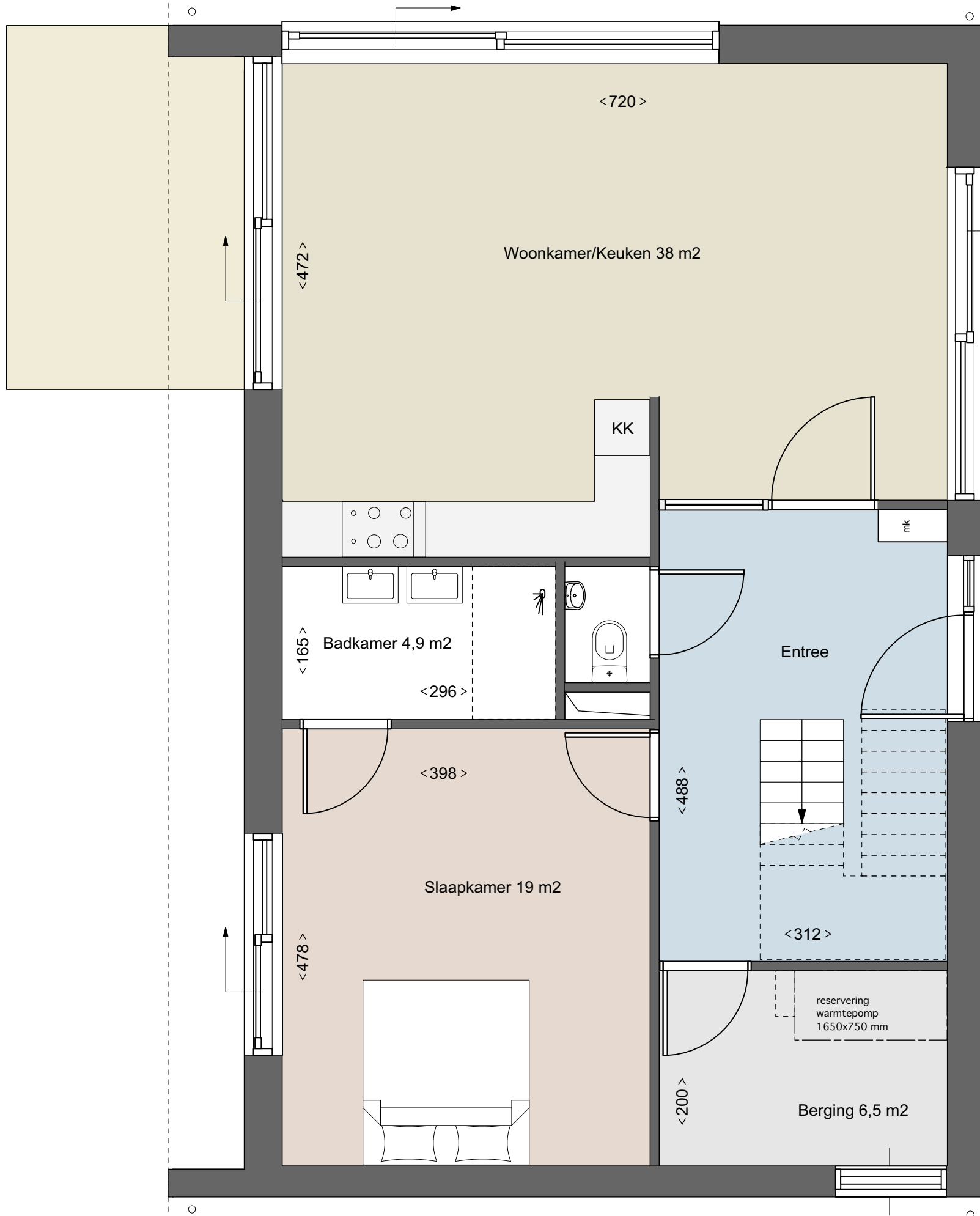
4C living Lansingerland - vrijstaande woning type 9 - slapen begane grond plattegrond begane grond
