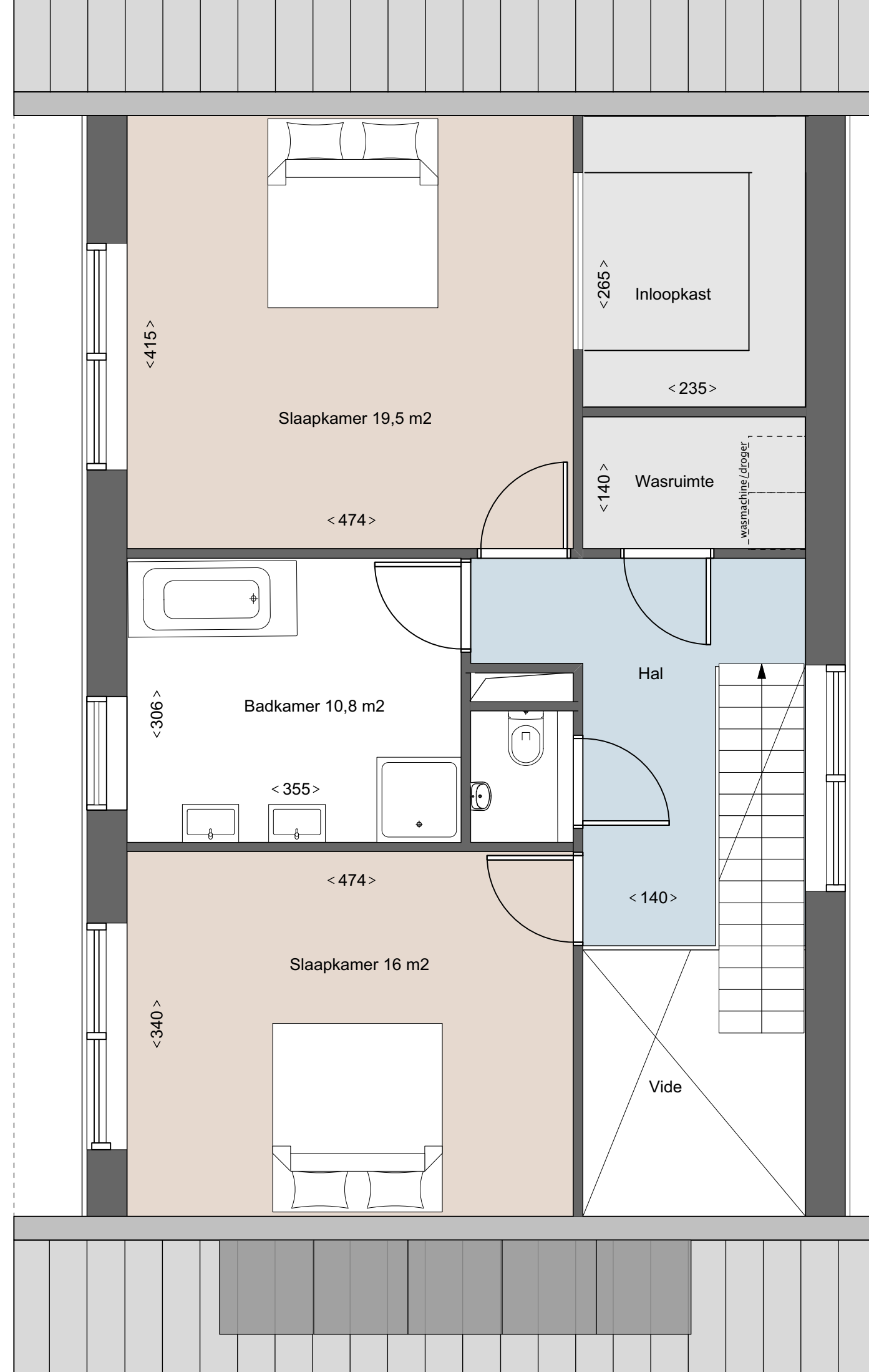
4C living Lansingerland - vrijstaande woning type 1 plattegrond verdieping
