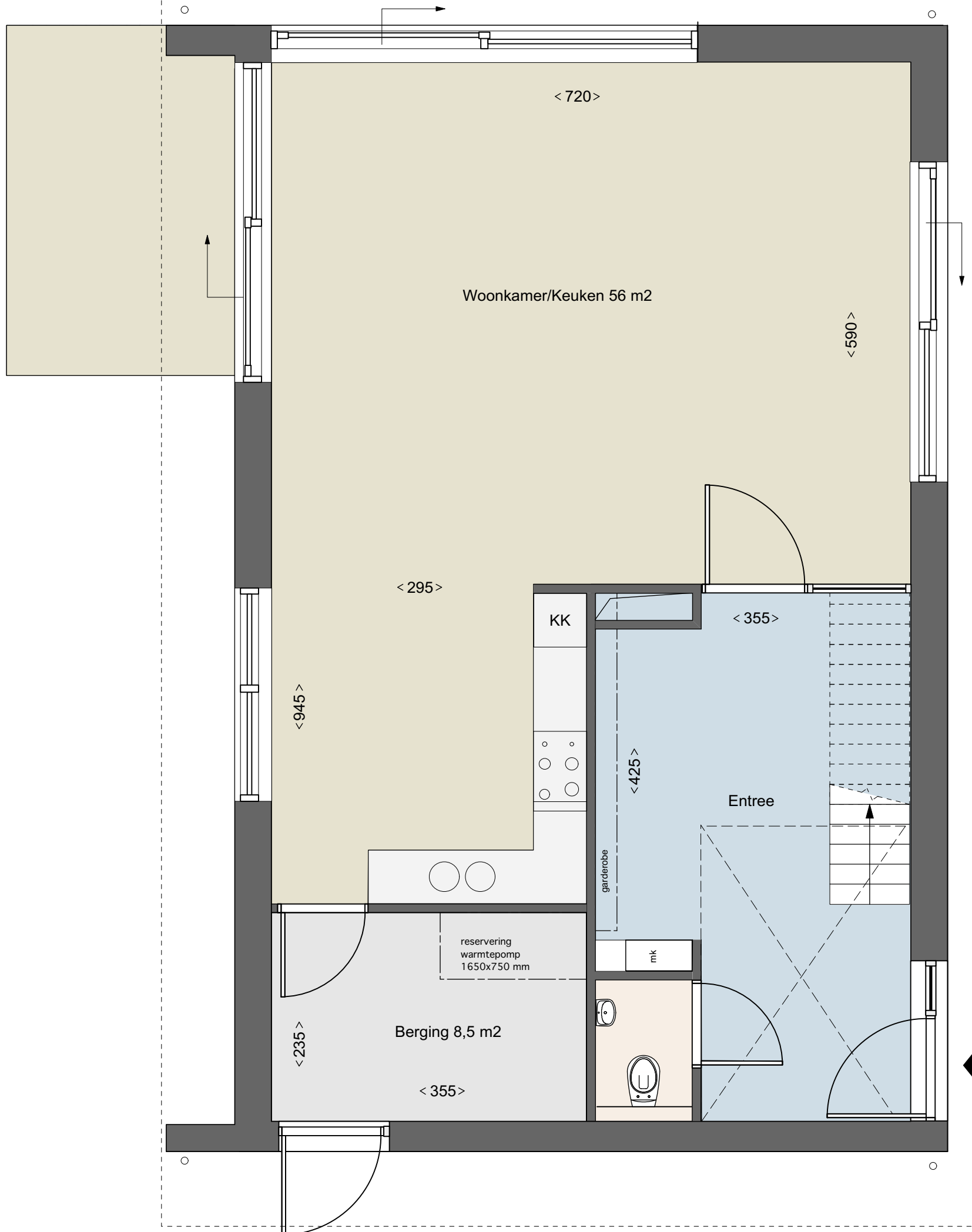
4C living Lansingerland - vrijstaande woning type 1 plattegrond begane grond
